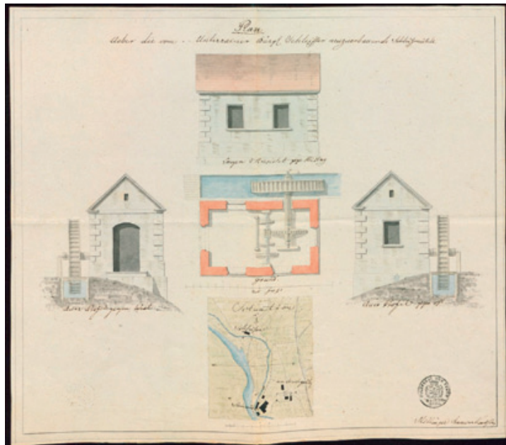
Archivalie des Monats September: Plan über die vom Unterrainer Schleifer neuzeubauende Schleifmühle, 1824, StadtA Wasserburg a. Inn, II485. Planzeichner: Millinger.
